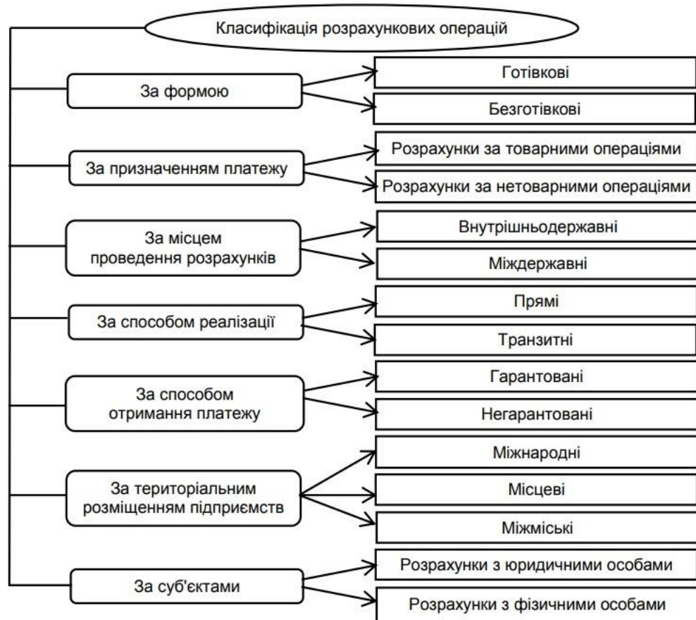
Рис. 1.4. Класифікація розрахунків
