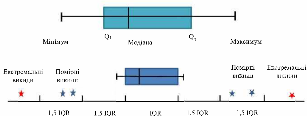
Рис. 2.9. Основні характеристики ящикової діаграми
