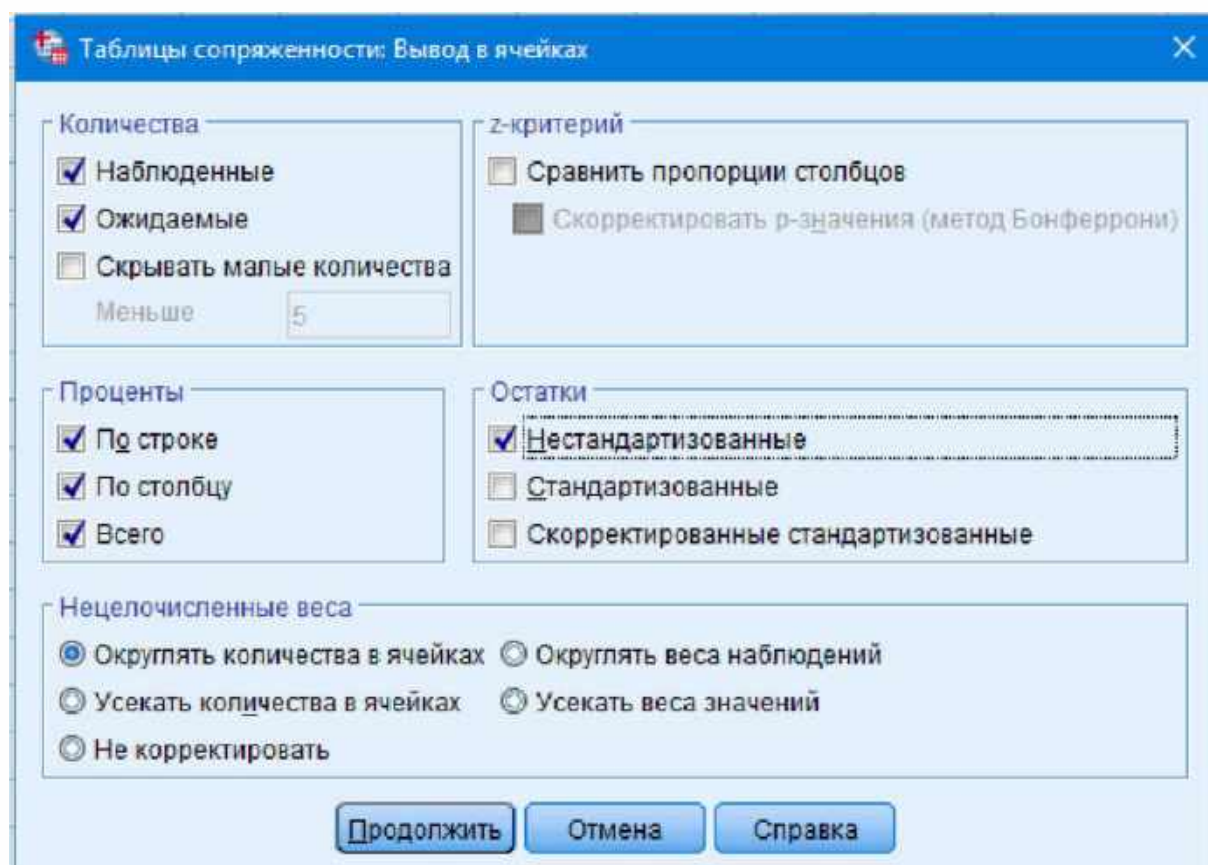
Рис. 4.18. Діалогове вікно SPSS
