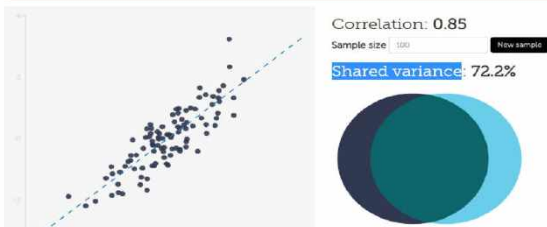
Рис. 5.3. Візуалізація сильної позитивної кореляції
