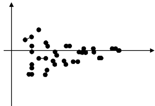
б) гетероскедастичність
