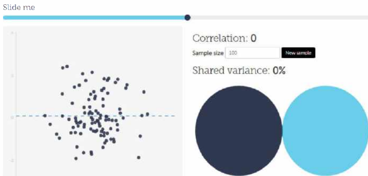
Рис. 5.5. Візуалізація нульової кореляції
