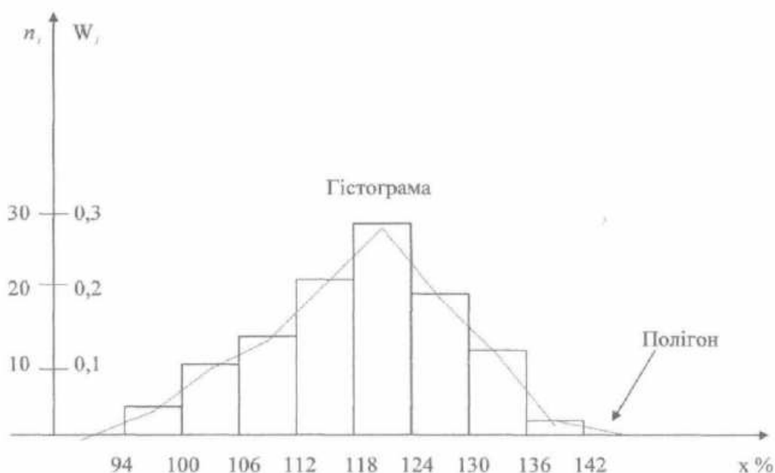
Рис. 2.4. Гістограма продуктивності праці одного робітника механічного цеху
