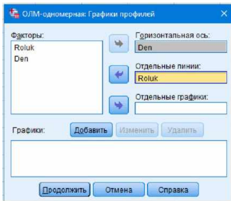
Рис. 4.8. Діалогове вікно SPSS
