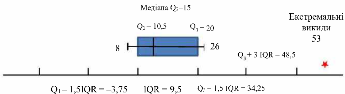
Рис. 2.10. Аналіз ряду спостереження за допомогою ящикової діаграми
