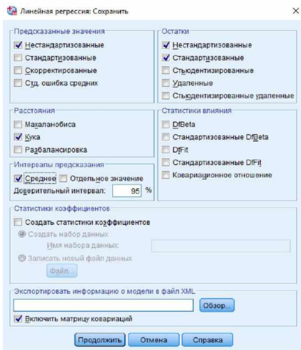
Рис. 6.11. Аналіз залишків
