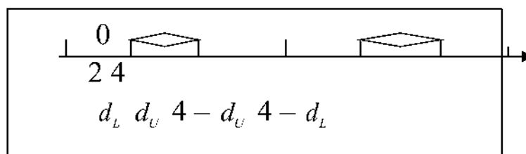
Рис. 6.14. Графічне використання тесту Дарбіна-Уотсона
