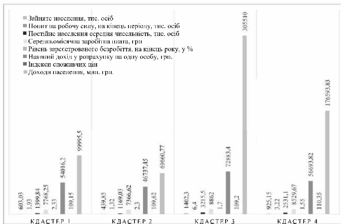
Рис. 2. Діаграма центрів кластерів
