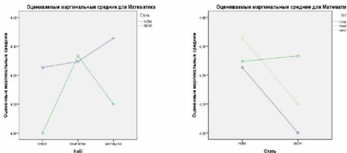
Рис. 4.15. Маргінальні середні величини для математики за статтю і хобі
