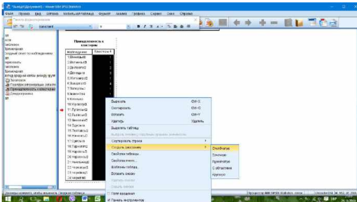
Рис. 7.7. Побудова діаграми
