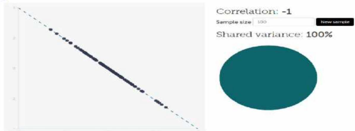
Рис. 5.2. Візуалізація чіткої негативної кореляції
