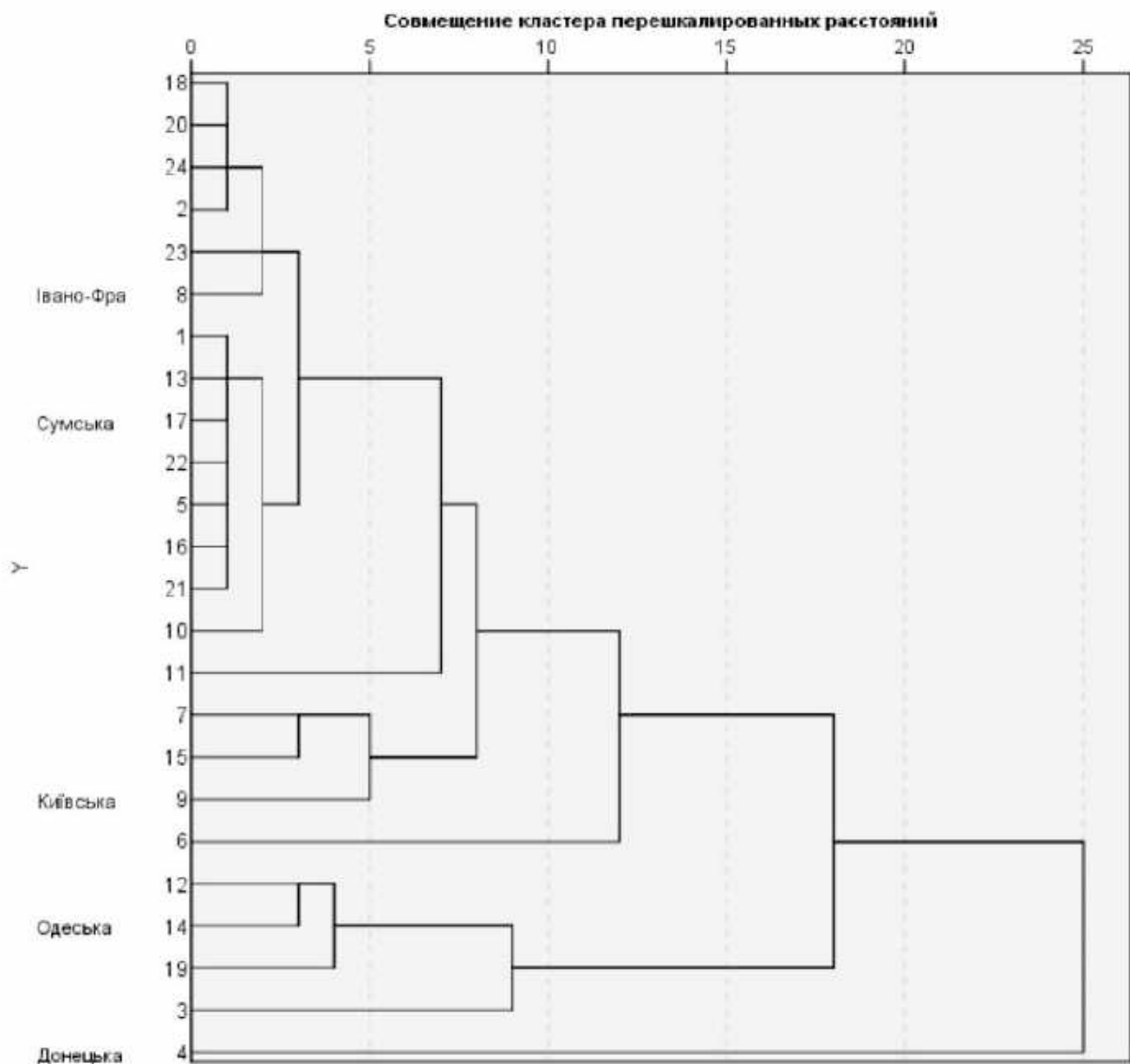
Рис. 7.9. Дендрограма ієрархічної кластеризації
