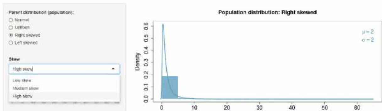
Рис. Високе (high) правостороннє відхилення (skew) генеральної сукупності
