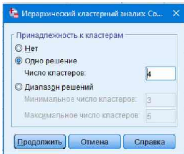
Рис. 7.6. Збереження ієрархічної кластеризації
