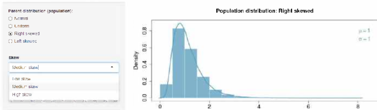
Рис. Середнє (medium) правостороннє відхилення (skew) генеральної сукупності
