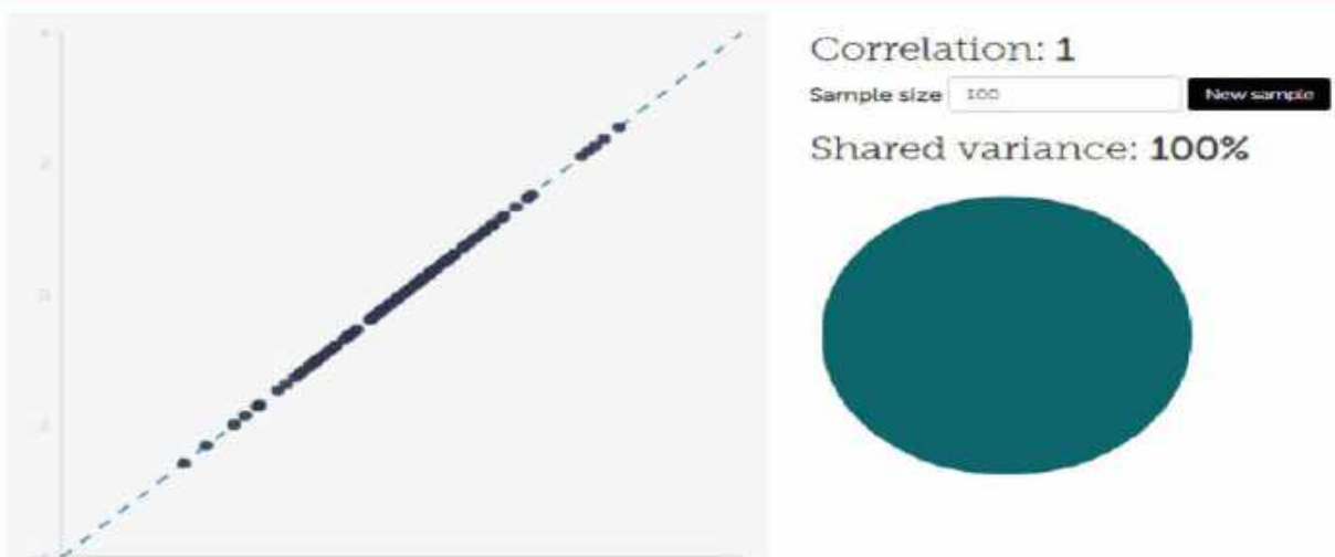
Рис. 5.4. Візуалізація чіткої позитивної кореляції
