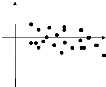
а) гомоскедастичність
