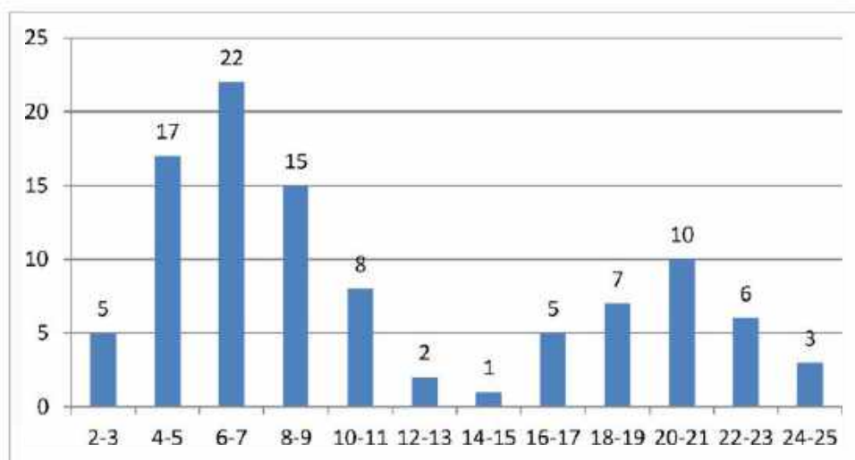
Рис. 2.6. Розподіл відпочиваючих на морі за кількістю днів
