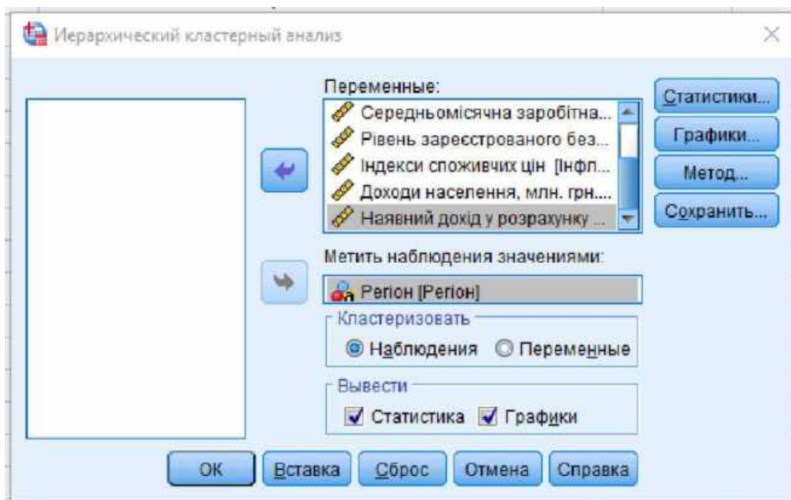
Рис. 7.2. Внесения параметров для проведения иерархической кластеризации
