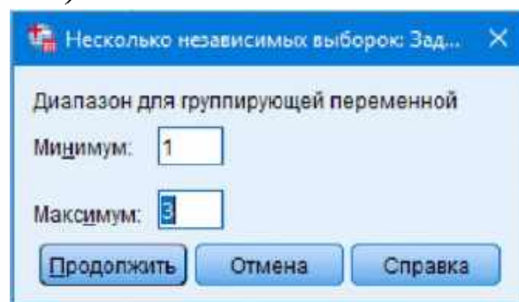
Рис. 3.19. Діалогове вікно SPSS
