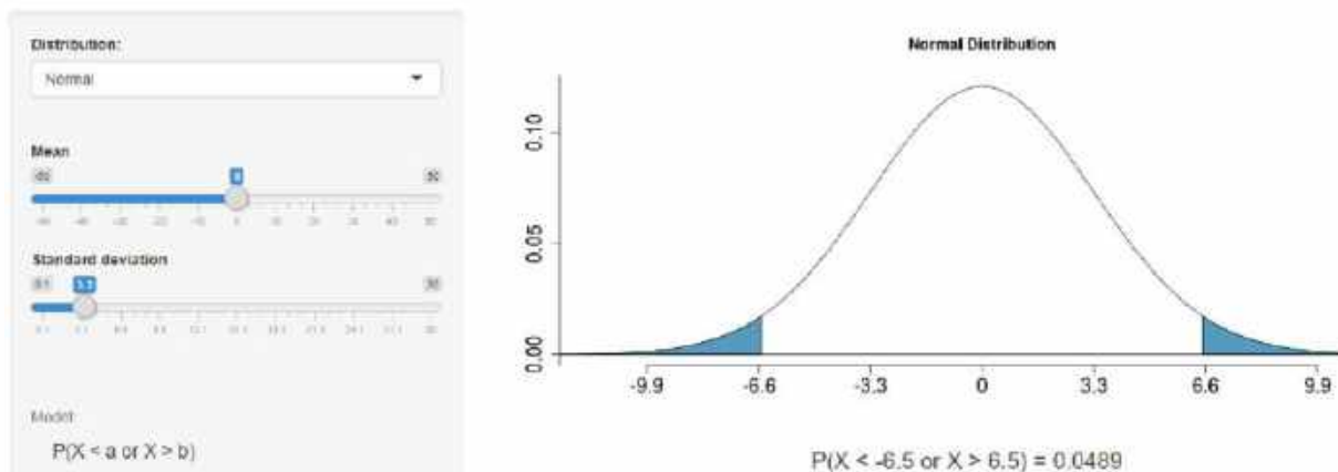
Рис. 3.2. Нормальний розподіл
