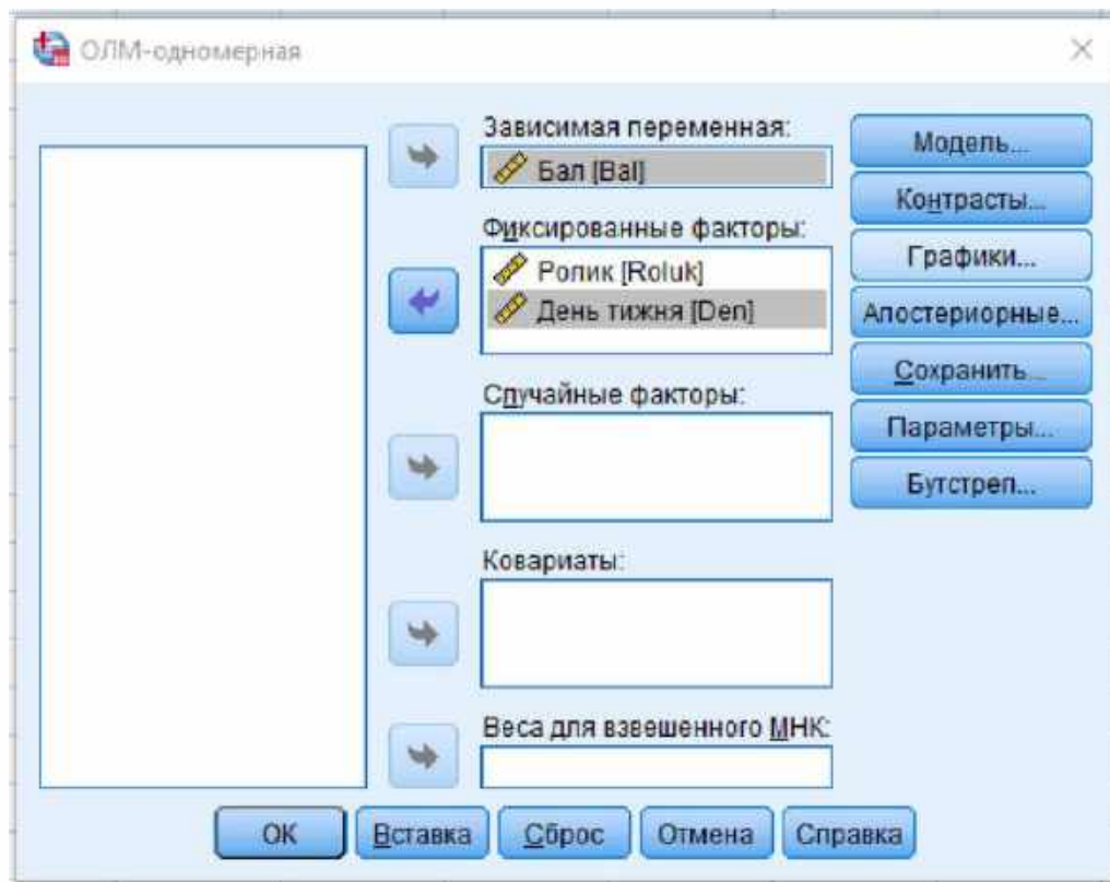
Рис. 4.7. Діалогове вікно SPSS
