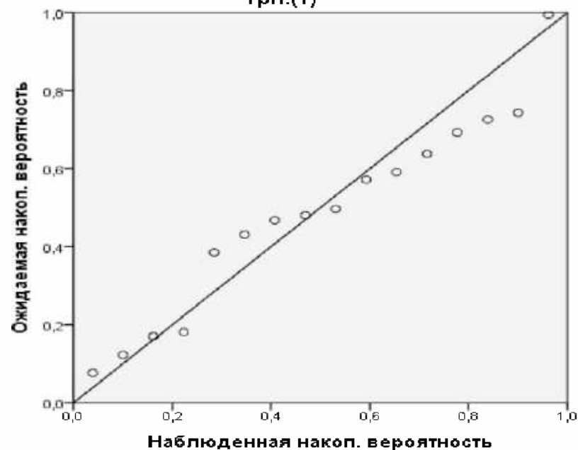
Рис. 6.15. Графік нормального розподілу стандартизованих залишків моделі
