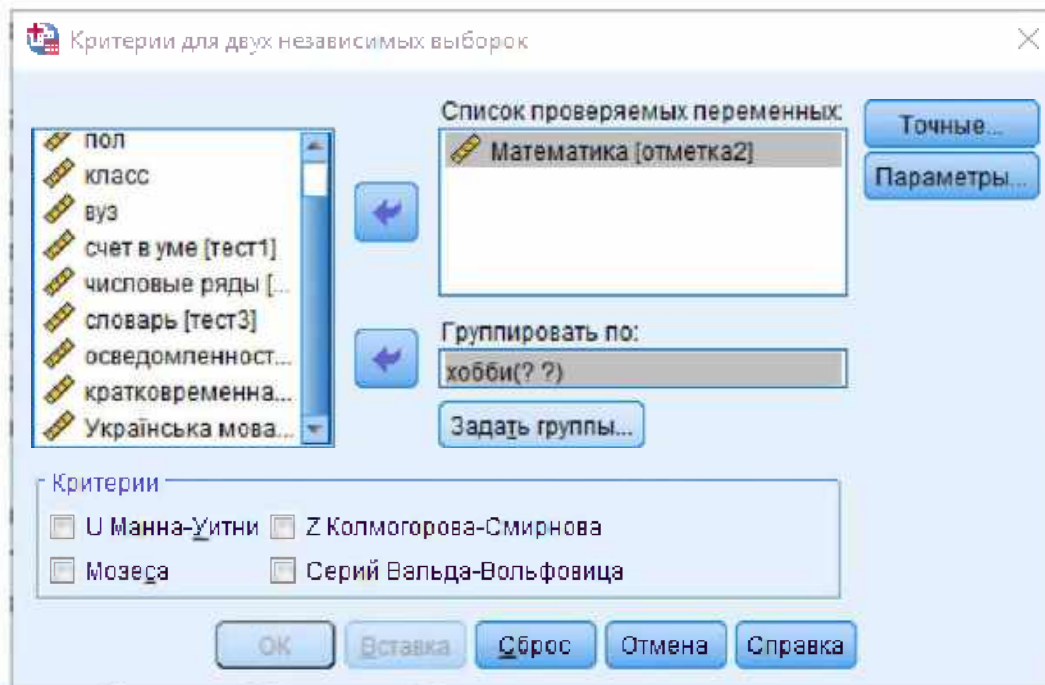
Рис. 3.21. Діалогове вікно SPSS
