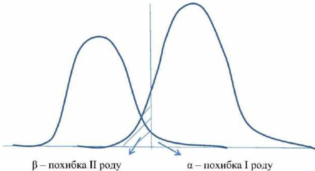
Рис. 3.1. Візуалізація похибки першого і другого роду
