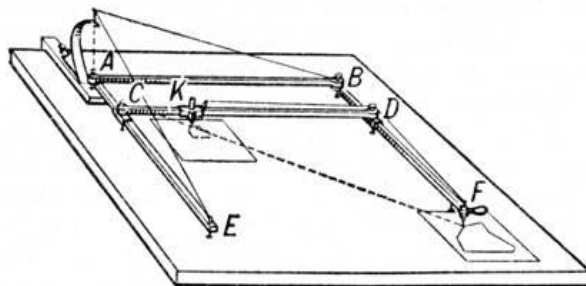
Рис. 19. Схема пантографа
