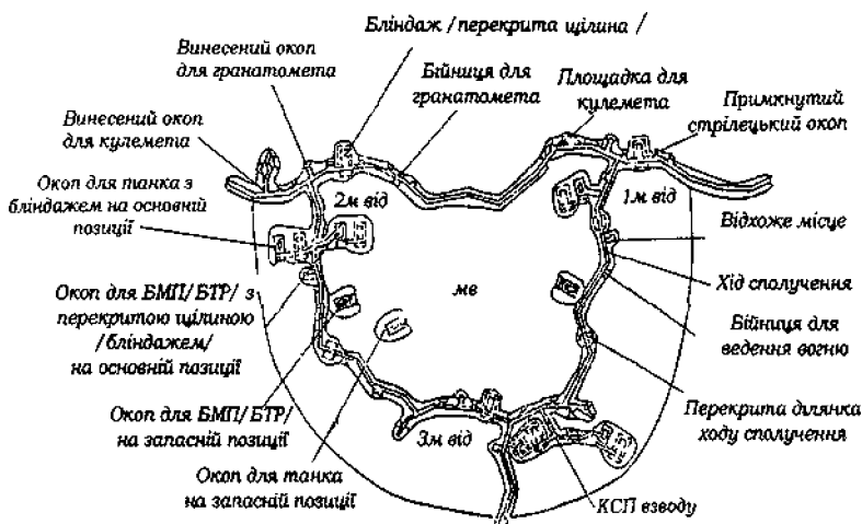
Рис. 2.3. Фортифікаційне обладнання опорного пункту взводу першого ешелону роти
