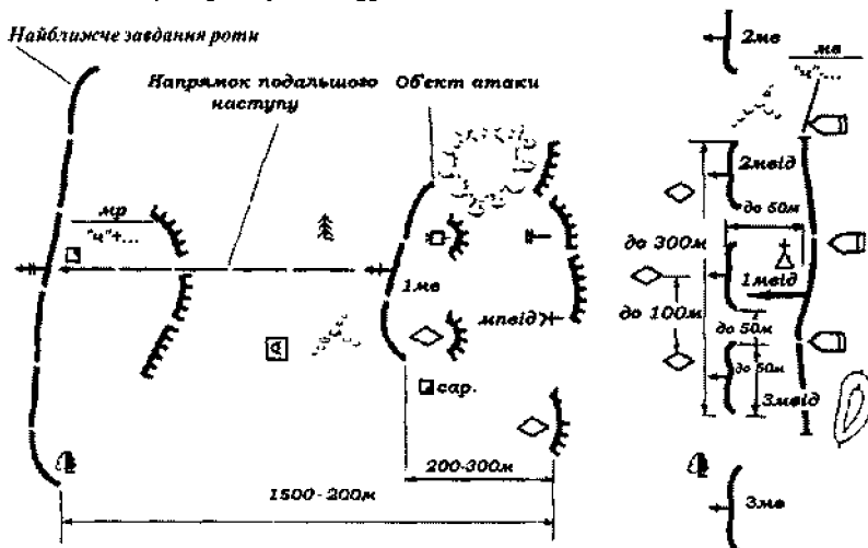
Рис. 3.1. Бойовий порядок та бойові завдання взводу в наступі
